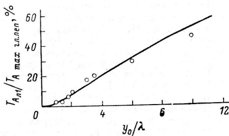
Рис. 9. Расширение главного лепестка д. н. в зависимости от выноса y_0/\lambda .
