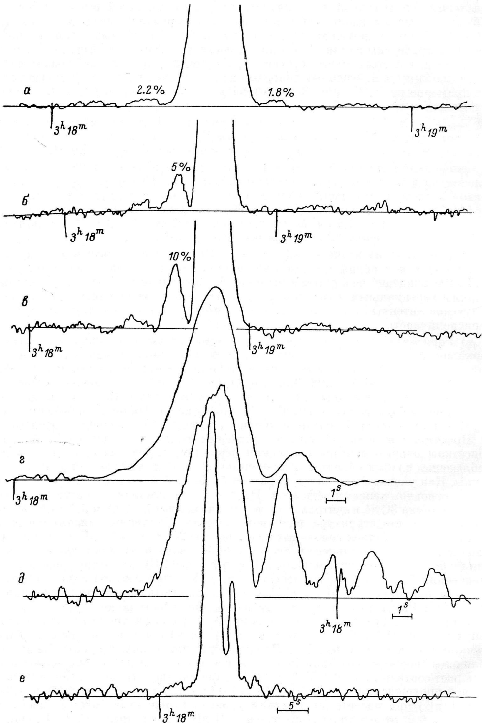
Рис. 7. Кривые прохождения источника ЗС 84 при различных выносах облучателя y_0/\lambda .
