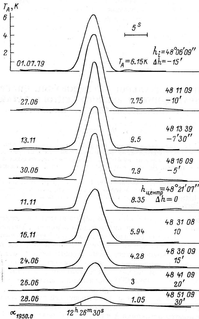
Рис. 1. Кривые прохождения источника ЗС 273 на волне \lambda=8.2 см в различных горизонтальных сечениях h_i (постоянная времени \tau=0^s.2 , калибровка производилась с помощью генератора шума ГШ=1.05 К.
